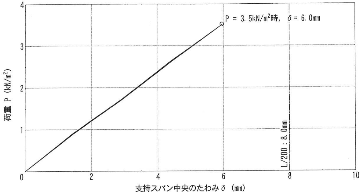
図3 荷重-たわみ曲線
