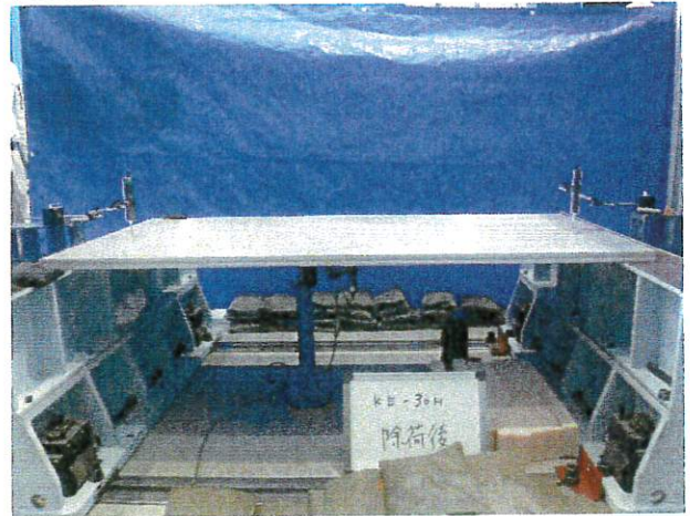
写真2 試験体状況 除荷後 ・異状なし
